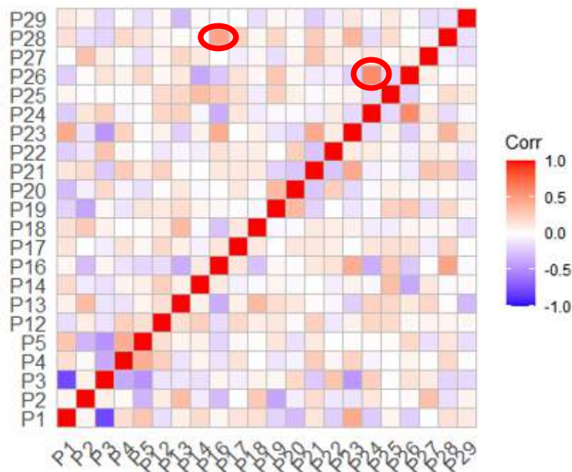
Figura N°1: Matriz de correlación de R.
